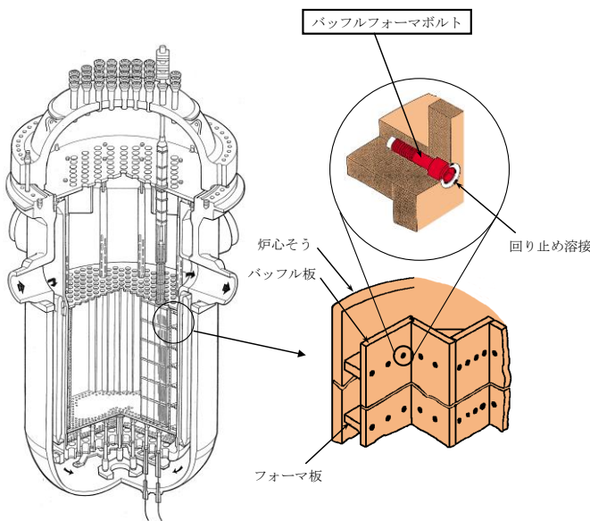
図 1.2.1-1 バッフルフォーマボルト
