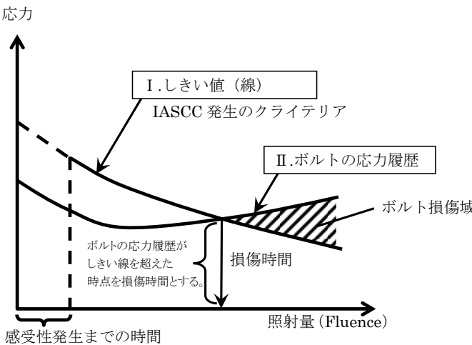
図 2.1.3-1 IASCC 損傷評価によるバッフルフォーマボルトの損傷時間の考え方
