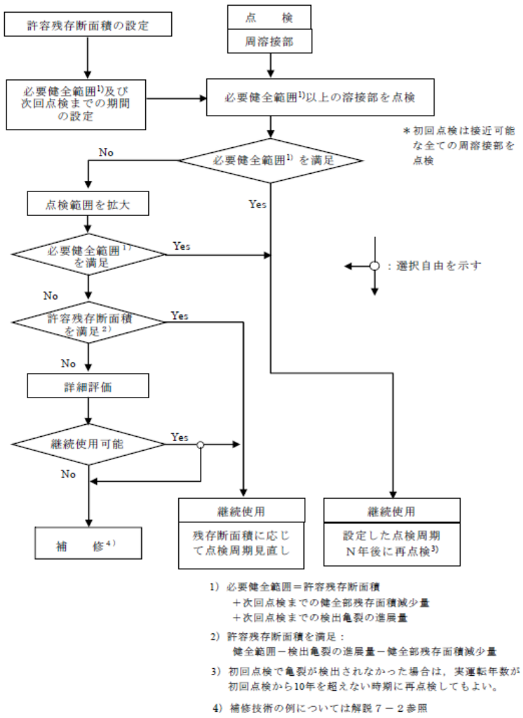
図 4-2 H1, H2 溶接線の点検の考え方
