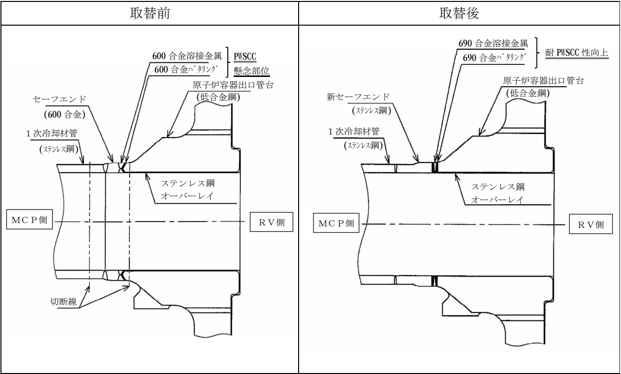
図 -1 施工前後の構造図
