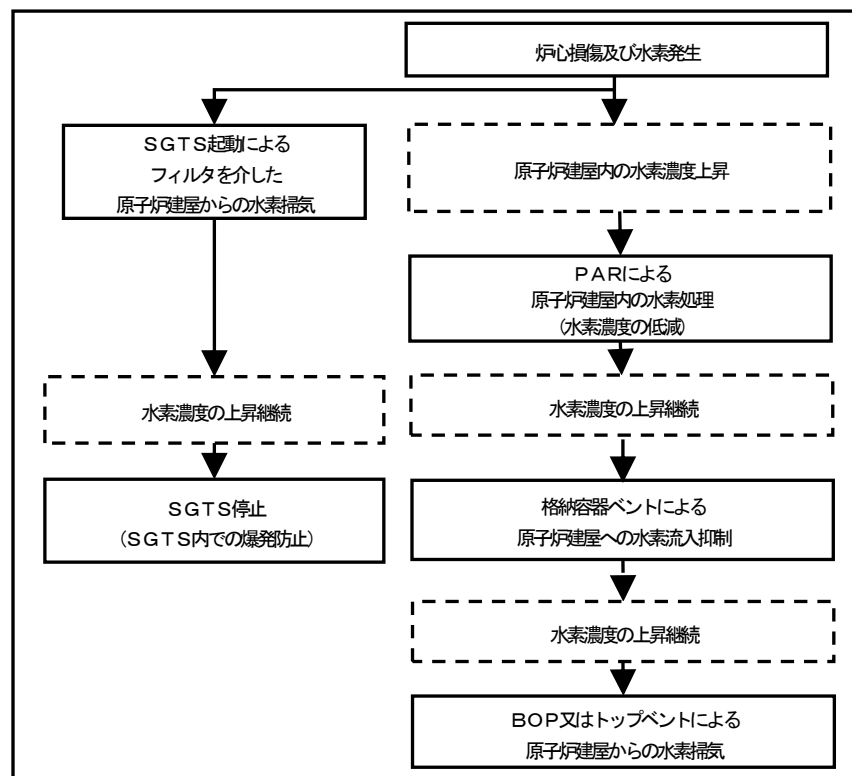
【新規規制基準対応を踏まえたAMGのフローの例】
