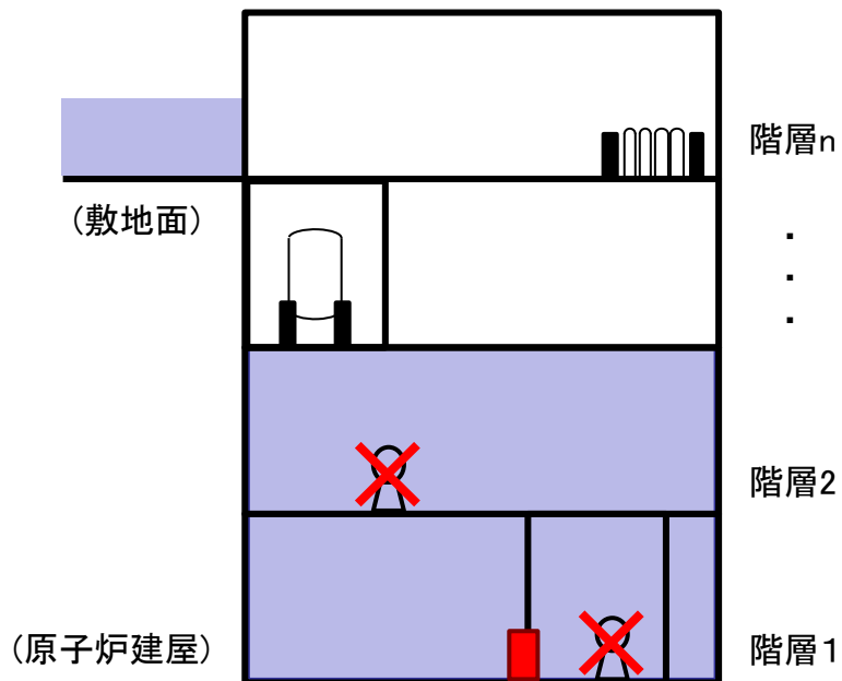
図2 建屋内浸水のイメージ（階層2より下部が浸水した場合）
