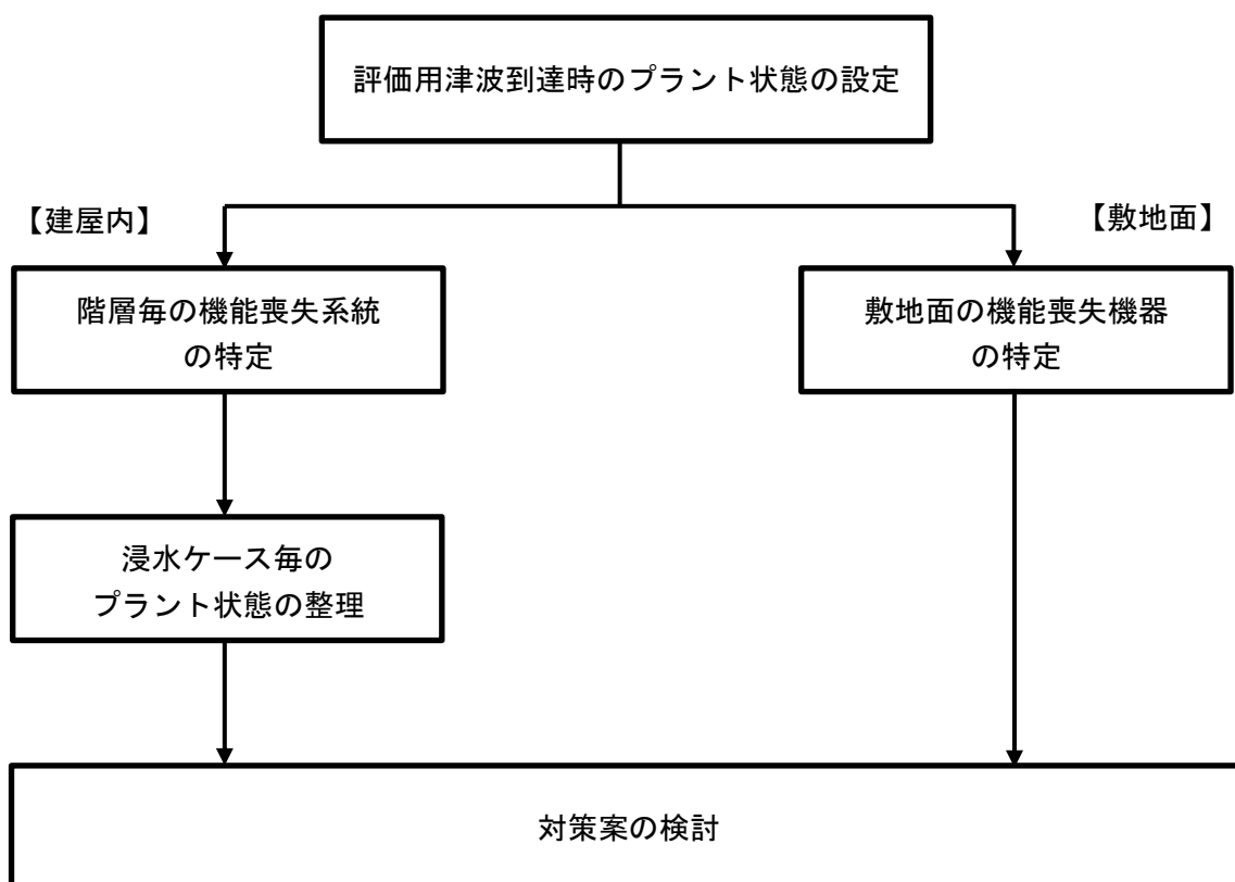
図 3 津波評価の評価フロー
