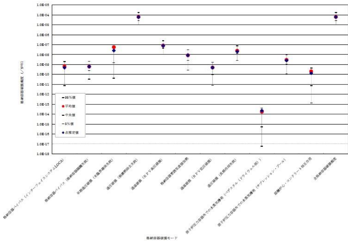
図 1-1 内的事象レベル 1.5PRA 評価結果 (Mark-I 改)
