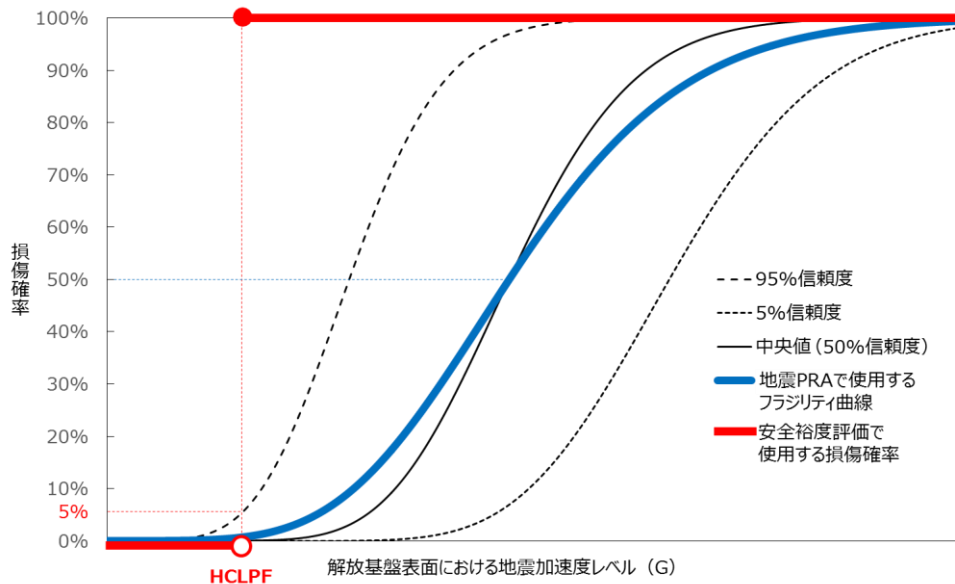
図1 地震に係る安全裕度評価と地震 PRA 評価における機器の損傷確率のイメージ
