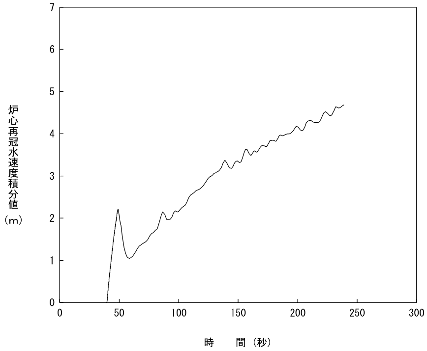
图4.5.1-6 炉心再冠水速度積分値 (低温側配管兩端破断 CD=0.4)
