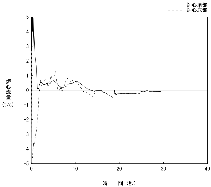
图4.5.1-3 炉心流量 (低温側配管兩端破断 CD=0.4)
