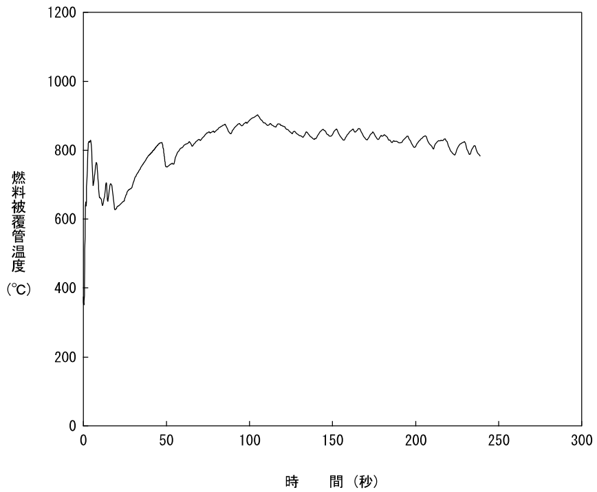
图4.5.1-7 燃料被覆管温度 (低温側配管兩端破断 CD=0.4)
