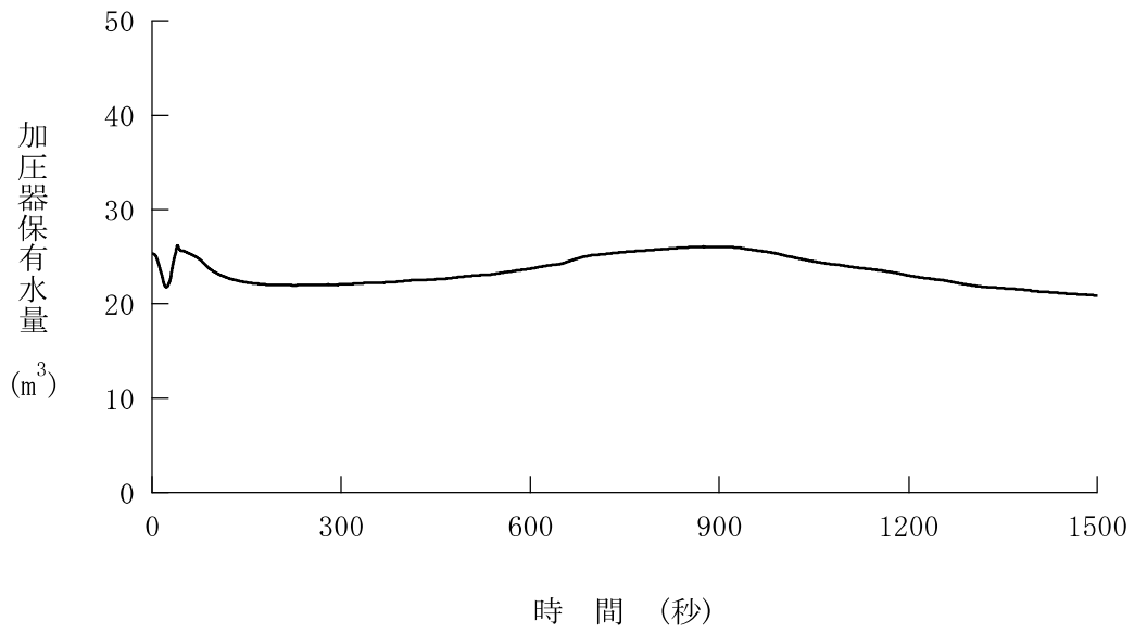
図 4.5.4.1-3 主給水管破断+ソフトウェア CCF (代表 3 ループプラント、加圧器保有水量)
