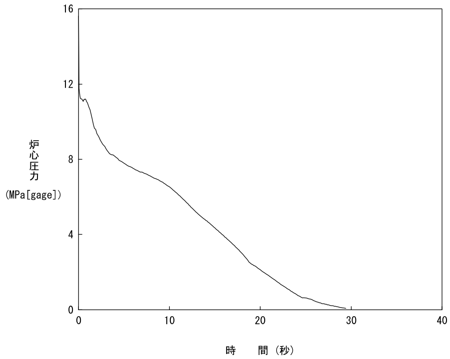
图4.5.1-2 炉心压力 (低温側配管兩端破断 CD=0.4)
