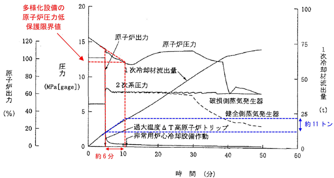
図 4.5.7.2-2 蒸気発生器伝熱管破損の添付書類十解析結果 (代表 4 ループプラント)
