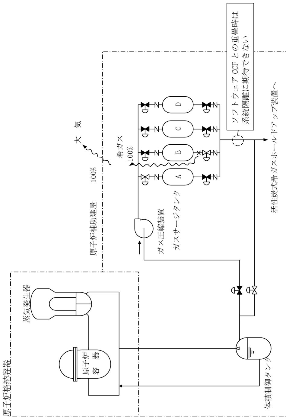
図 4.6.3-1 放射性気体廃棄物処理施設の破損時の放射能放出経路
