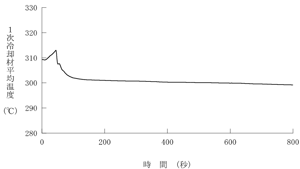
図 4. 4. 1. 2-4 主給水流量喪失+ソフトウェア CCF (代表 4 ループプラント、1 次冷却材平均温度)
