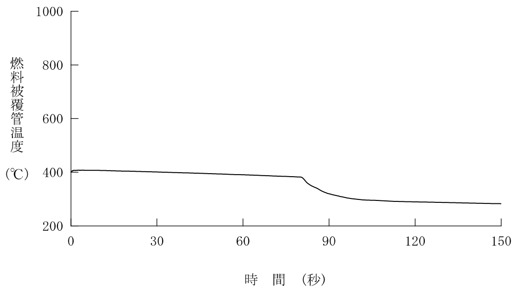
図 4. 5. 6. 1-7 制御棒飛び出し（サイクル初期高温全出力）＋ソフトウェア CCF （代表 3 ループプラント、燃料被覆管温度－MOX 燃料）
