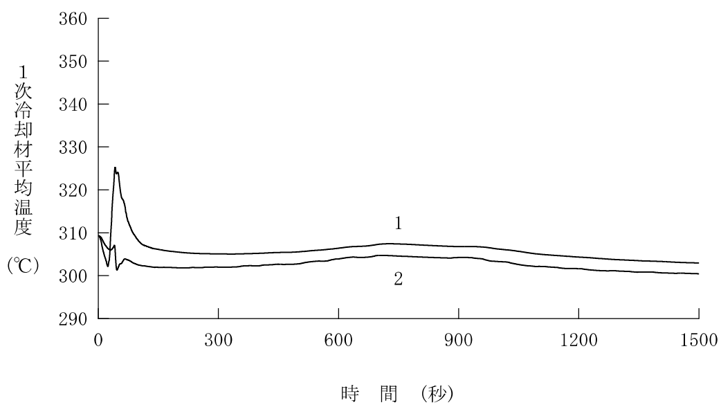
図 4. 5. 4. 2-4 主給水管破断+ソフトウェア CCF
