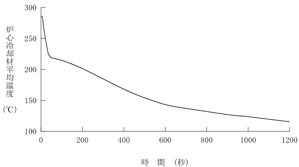
図 4. 5. 5. 1-2 主蒸気管破断+ソフトウェア CCF
