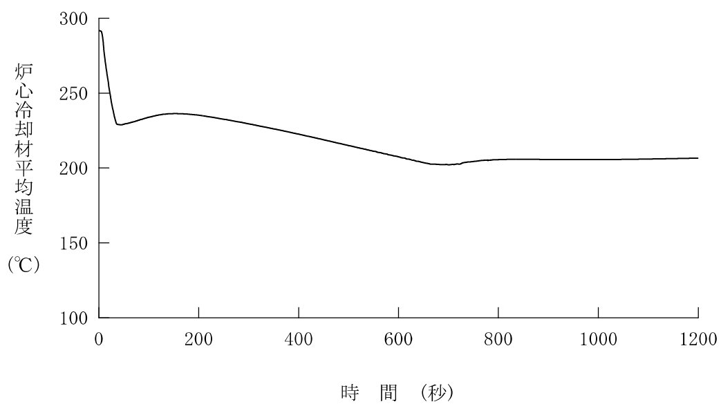
図 4. 5. 5. 2-2 主蒸気管破断+ソフトウェア CCF
