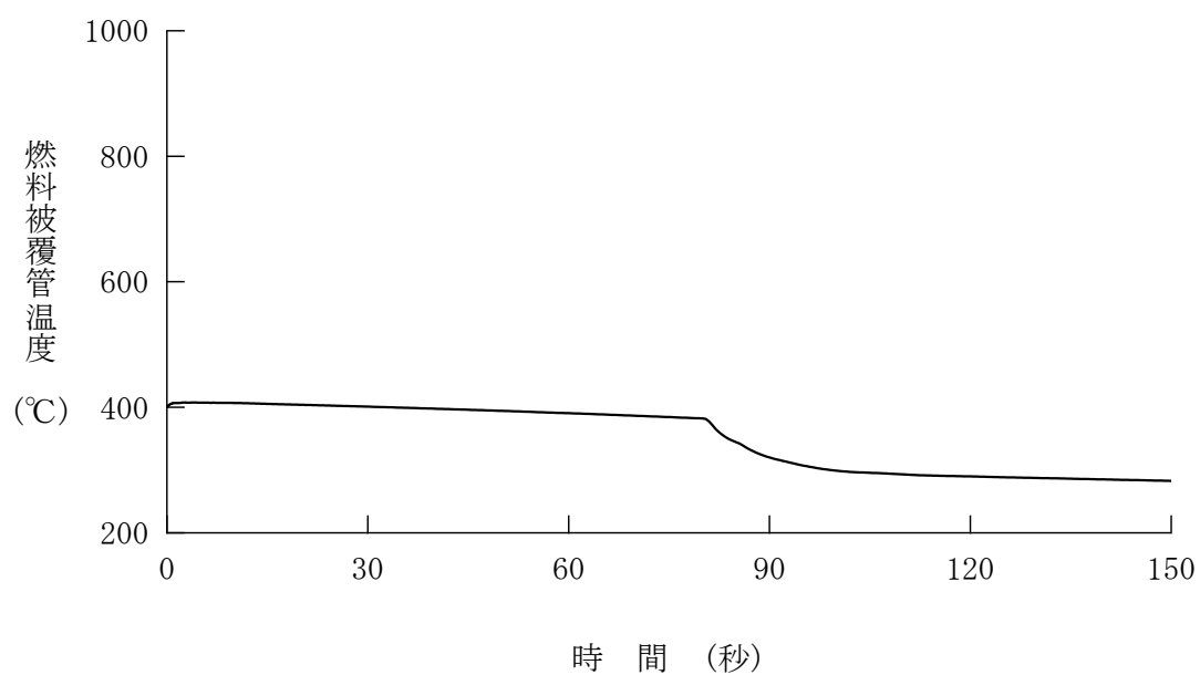
図 4.5.6.1-5 制御棒飛び出し（サイクル初期高温全出力）＋ソフトウェア CCF （代表 3 ループプラント、燃料被覆管温度－UO 2 燃料）
