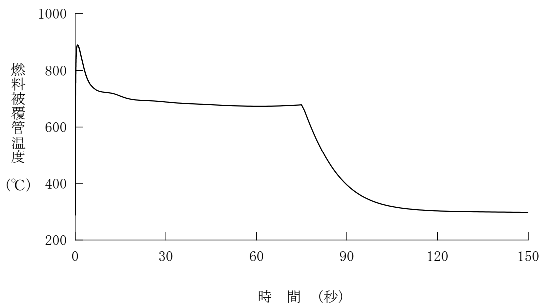
図 4.5.6.1-14 制御棒飛び出し（サイクル末期高温零出力）＋ソフトウェア CCF （代表 3 ループプラント、燃料被覆管温度－MOX 燃料）
