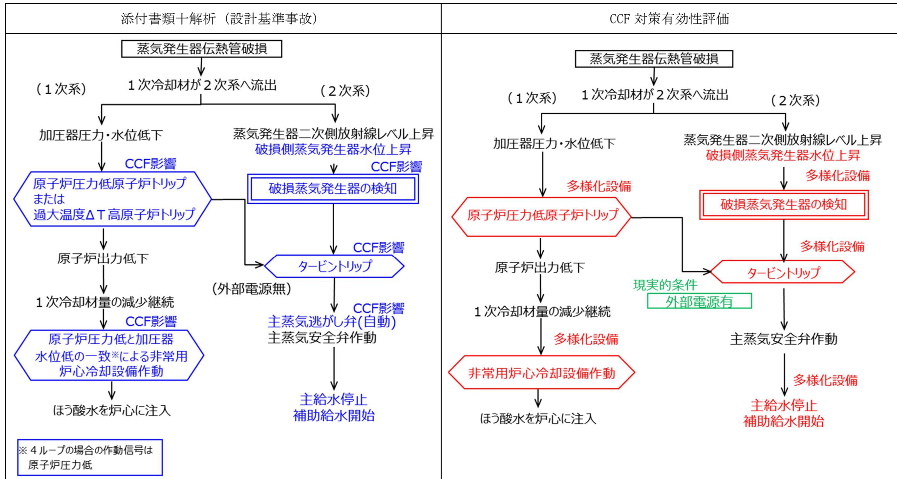
図 4.5.7-1 「蒸気発生器伝熱管破損」の事象進展（1）
