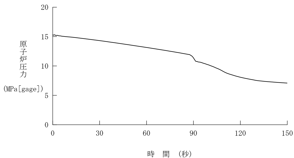
図 4.5.6.2-3 制御棒飛び出し（サイクル初期高温全出力）＋ソフトウェア CCF （代表 4 ループプラント、原子炉圧力）
