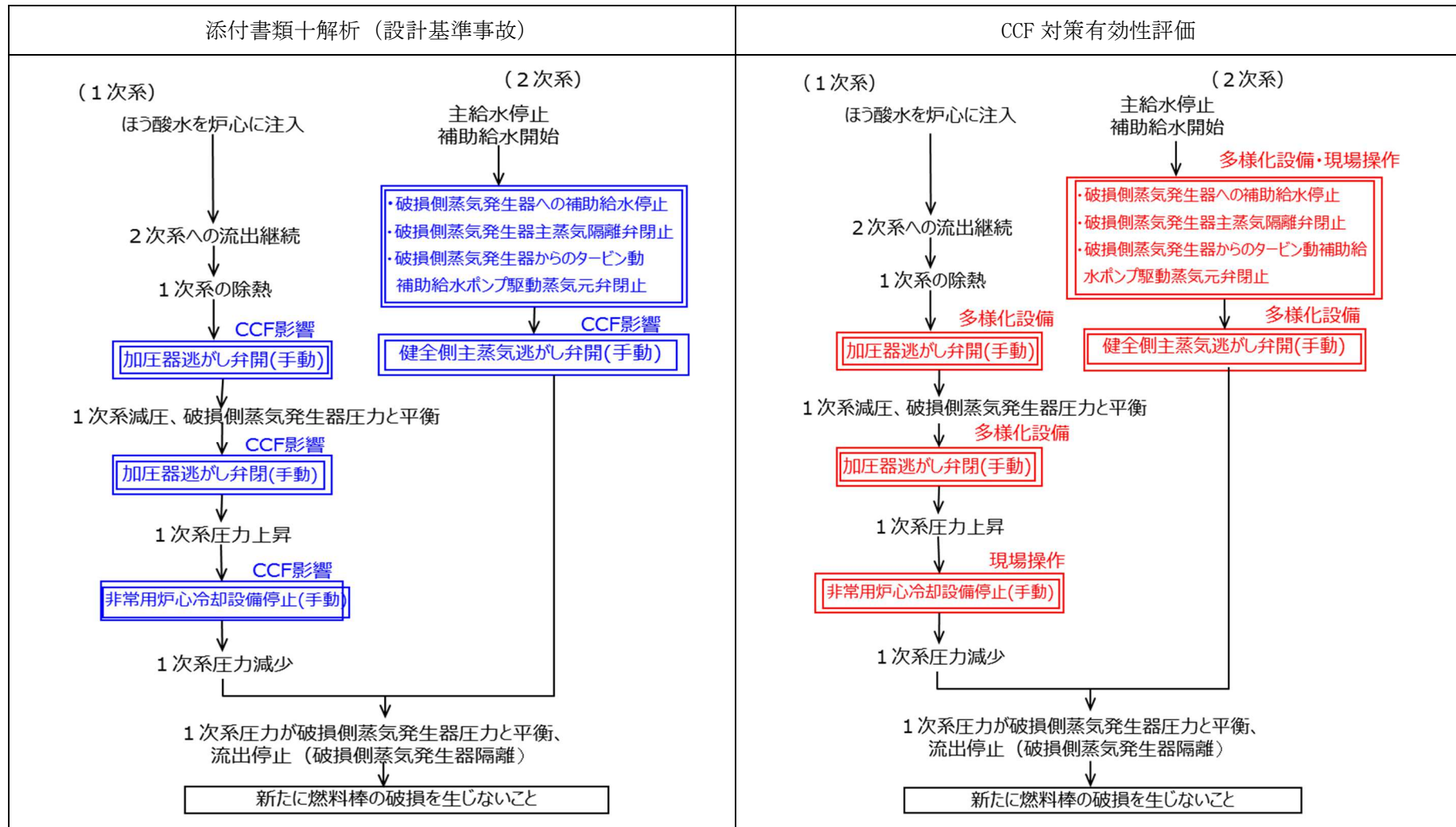
図 4.5.7-2 「蒸気発生器伝熱管破損」の事象進展（2）
