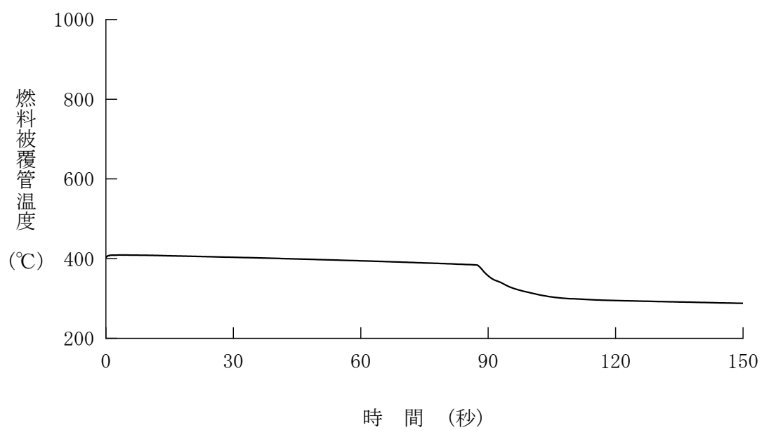
図 4. 5. 6. 2-5 制御棒飛び出し（サイクル初期高温全出力）＋ソフトウェア CCF （代表 4 ループプラント、燃料被覆管温度）
