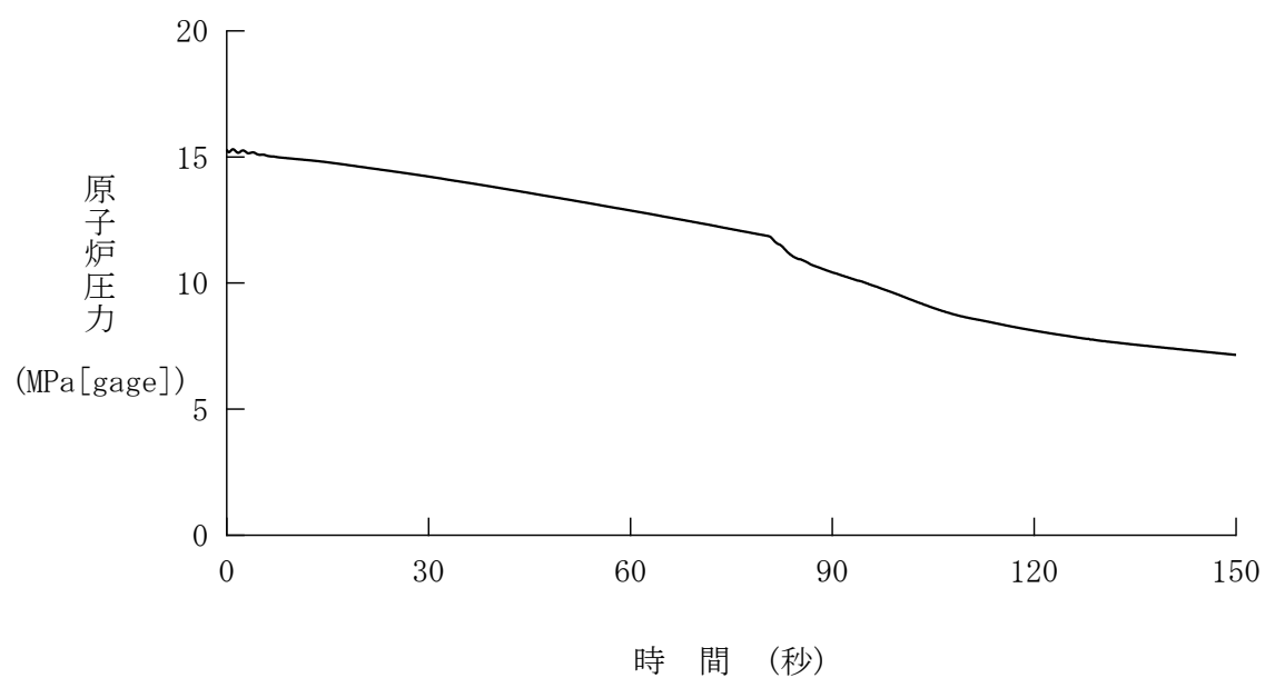
図 4.5.6.1-3 制御棒飛び出し（サイクル初期高温全出力）＋ソフトウェア CCF (代表 3 ループプラント、原子炉圧力)
