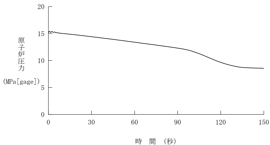
図 4.5.6.2-8 制御棒飛び出し（サイクル末期高温零出力）＋ソフトウェア CCF （代表 4 ループプラント、原子炉圧力）
