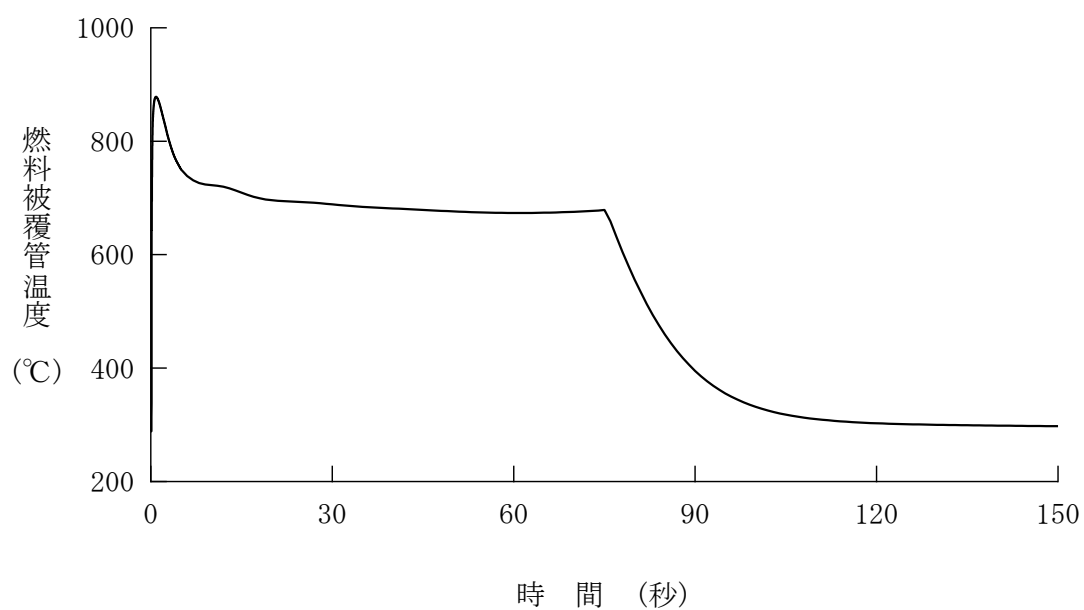
図 4.5.6.1-12 制御棒飛び出し（サイクル末期高温零出力）＋ソフトウェア CCF （代表 3 ループプラント、燃料被覆管温度－UO 2 燃料）
