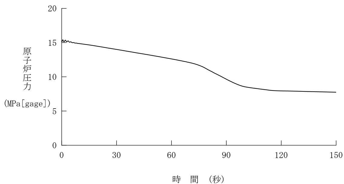
図 4.5.6.1-10 制御棒飛び出し（サイクル末期高温零出力）＋ソフトウェア CCF (代表 3 ループプラント、原子炉圧力)
