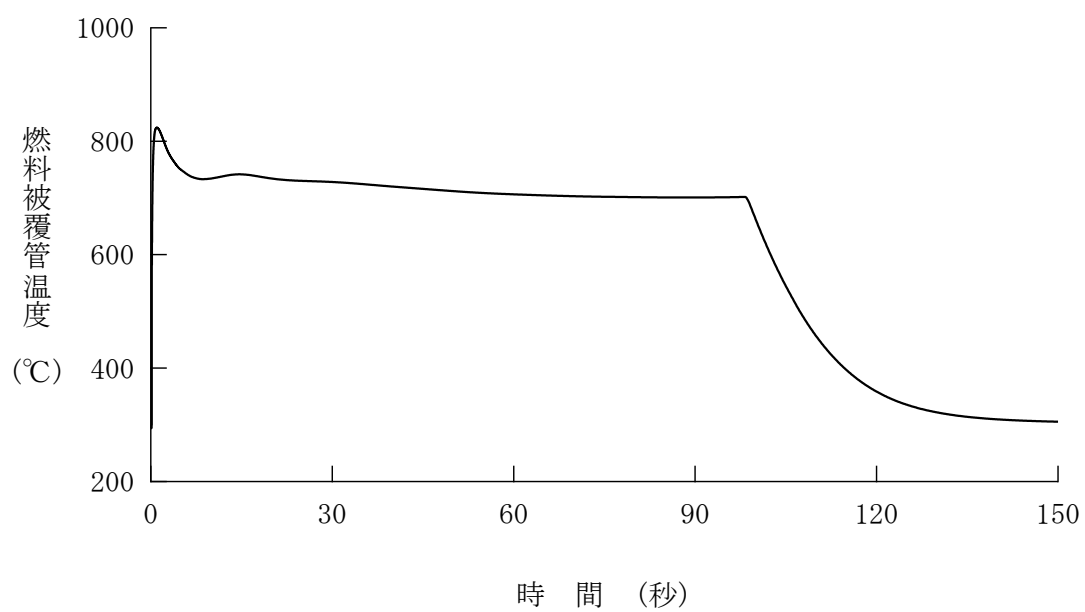
図 4.5.6.2-10 制御棒飛び出し（サイクル末期高温零出力）＋ソフトウェア CCF （代表 4 ループプラント、燃料被覆管温度）
