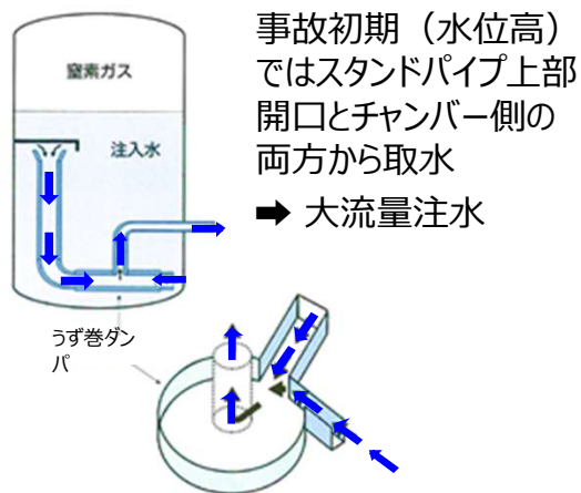
①大流量注水時
