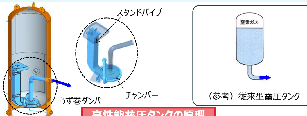
高性能蓄圧タンクの原理
