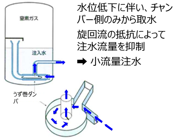
②小流量注水時
