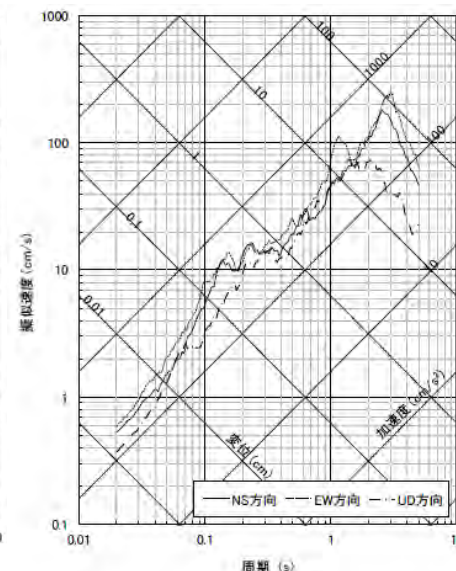
断層モデル波
