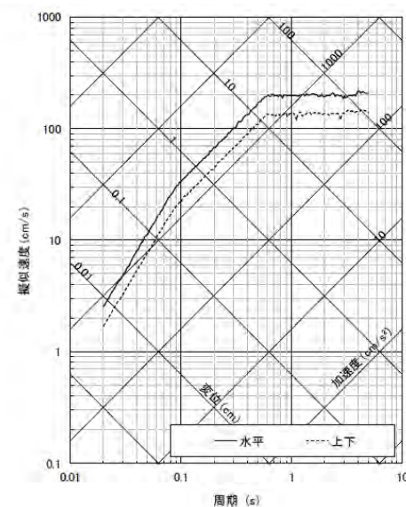
応答スペクトル波
