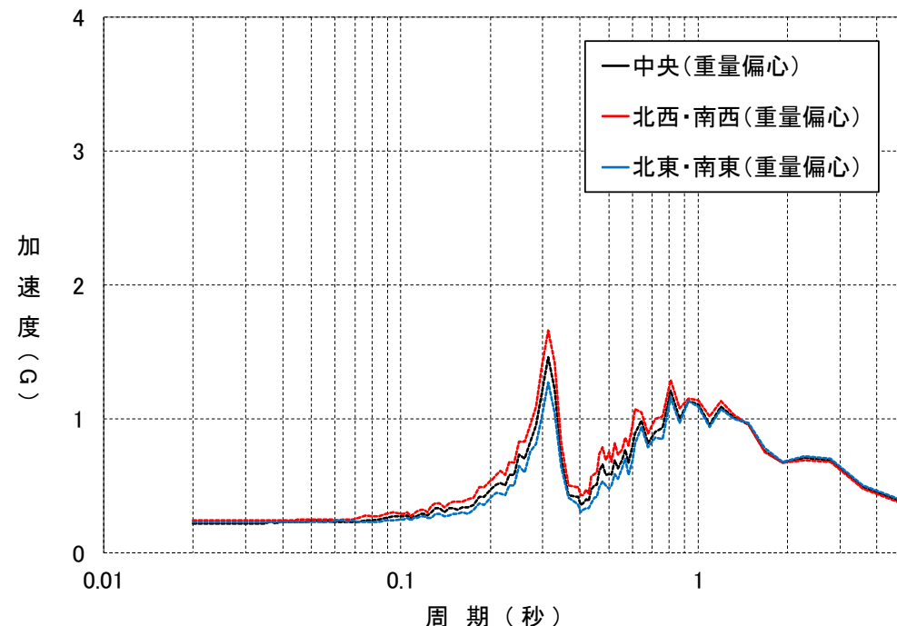
中央および4隅のNS方向の床応答スペクトル (減衰2.0%、スペクトル波NS単独同時入力)
