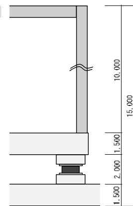
概略断面図
