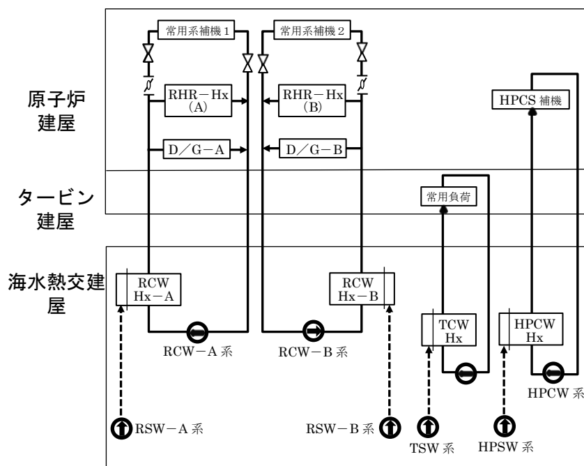
図3 中間型の補機冷却系（柏崎刈羽2～7，浜岡，女川，志賀，島根3）BWRの例
