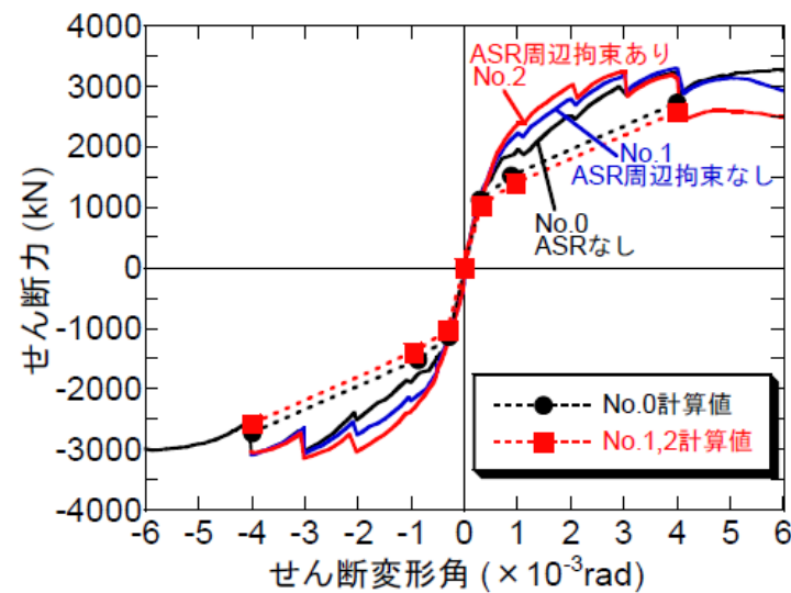
図7 復元力特性
