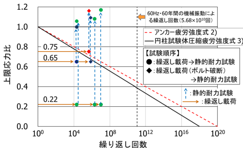
図2 S-N 曲線上における試験結果
