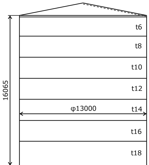
図 3 燃料取替用水タンク外形
